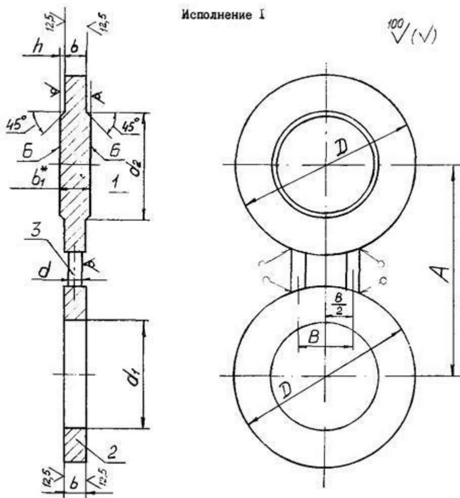
1 - заглушка; 2 - кольцо; 3 - вставка.
