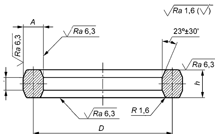
Рисунок 2 — Прокладки восьмиугольного сечения типа 2 для фланцев по ГОСТ 33259
