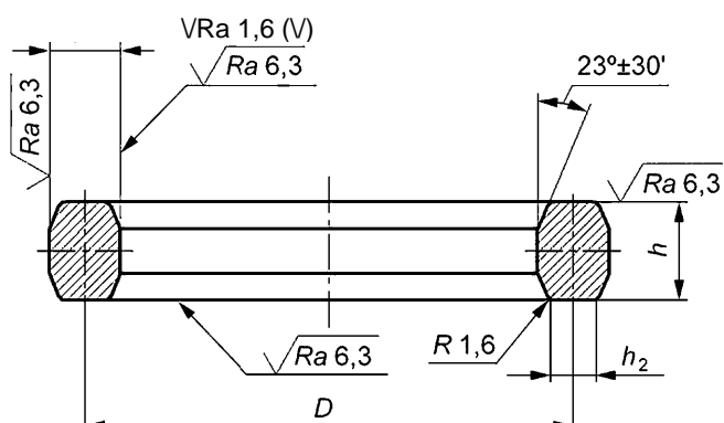
Рисунок 3 — Прокладки восьмиугольного сечения типа 2 для фланцев (см. [1])
