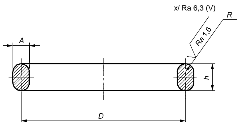
Рисунок 1 — Прокладки овального сечения типа 1 для фланцев по ГОСТ 33259 (см. также [1])
